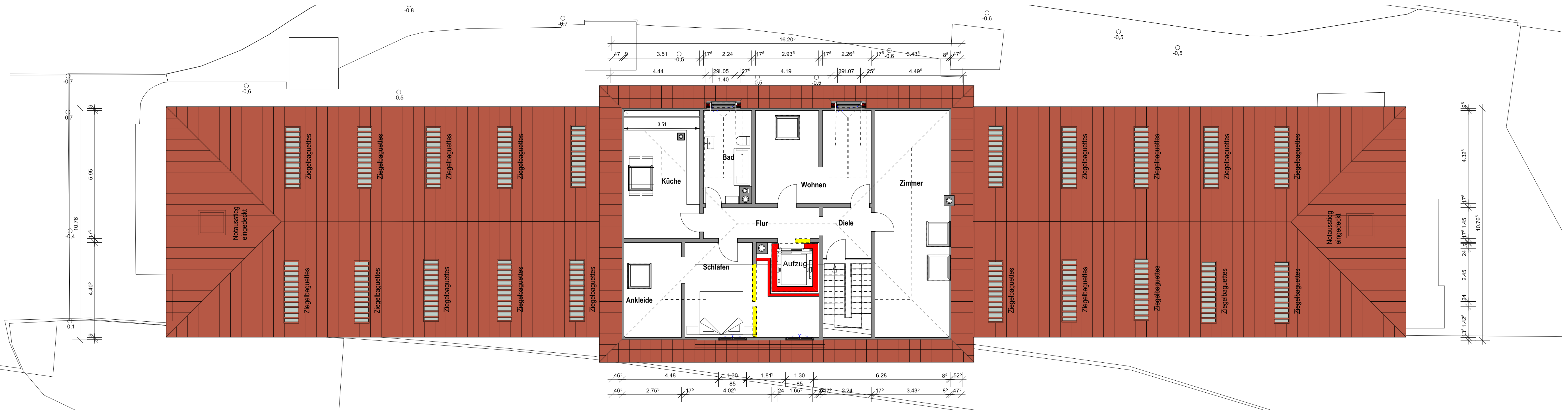
DACHGESCHOSS
